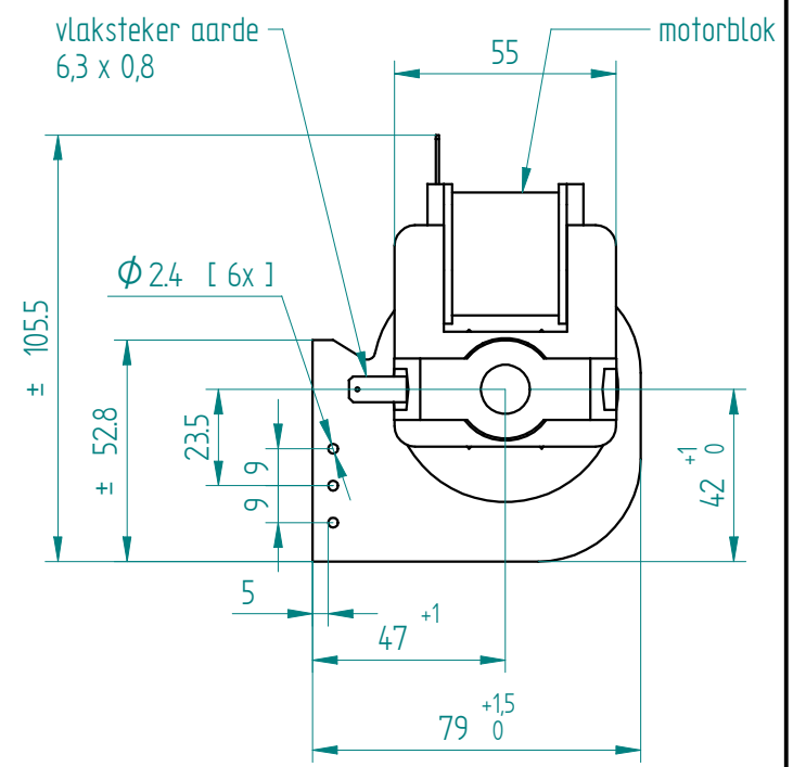
aanzicht motorblok zijde
